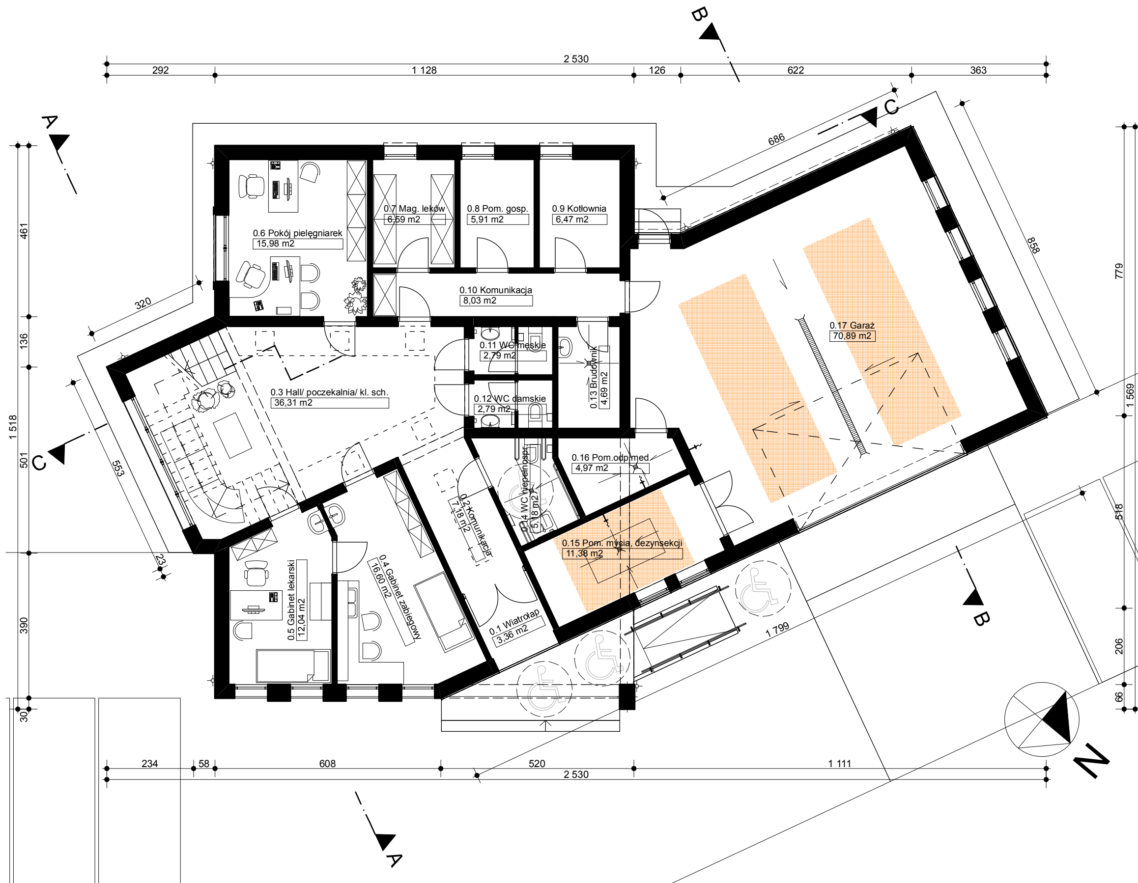
RZUT PARTERU 1:100
